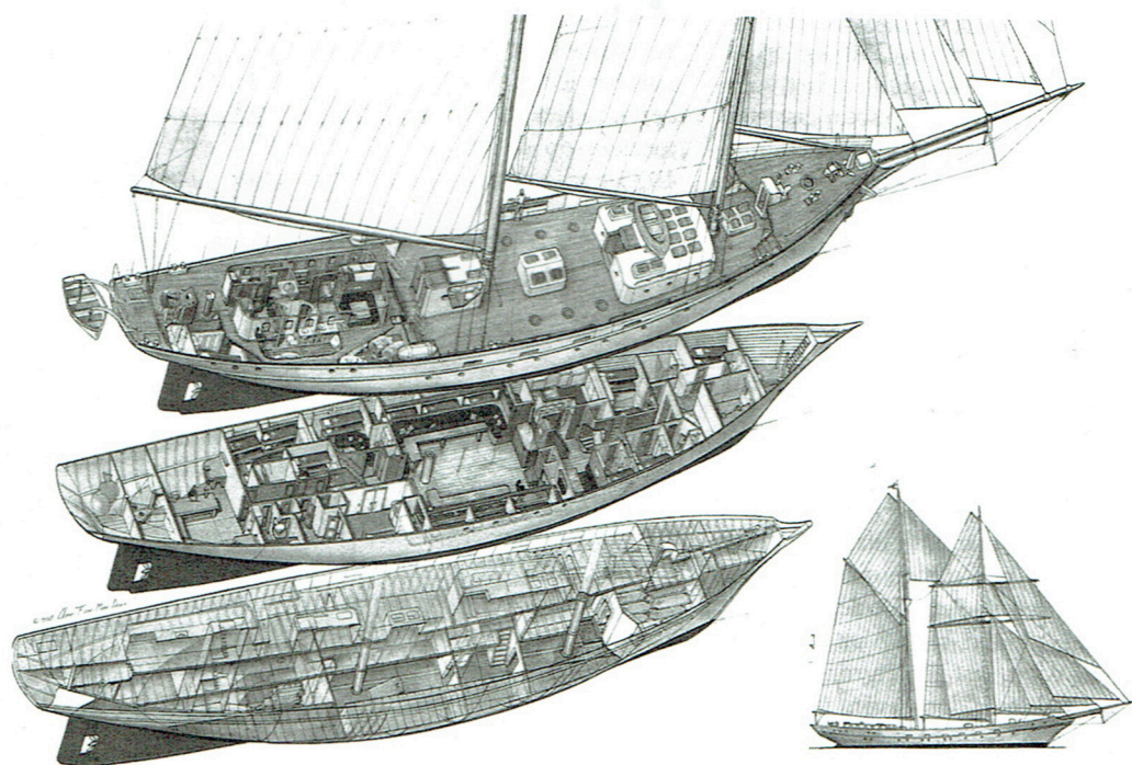
Onder: Artist impressions van de 46 m trainingschoener
